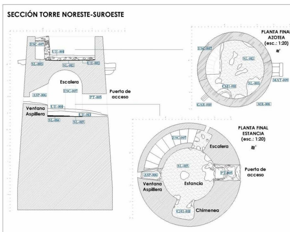
Sección de la Torre y planta de la Estancia y Azotea. Gespad al-Andalus S.L.U. 2010.
